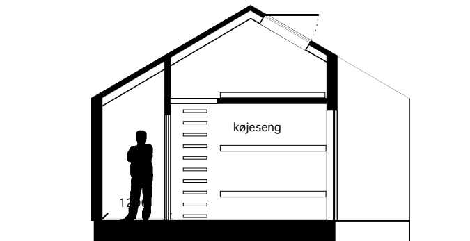
snit 1:100 børneværelse med adgang til hems med tagvindue.
