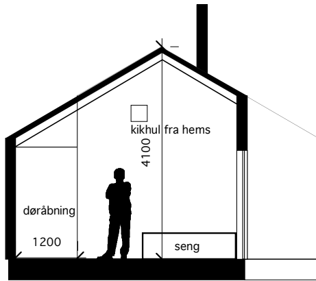
snit 1:100 sovoværelse
