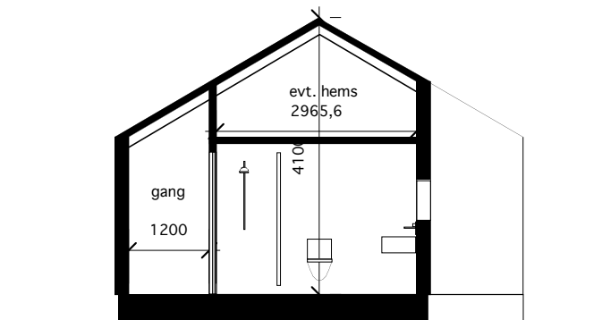
snit 1:100 badeværelse evt. hems over badeværelse med adgang fra værelse
